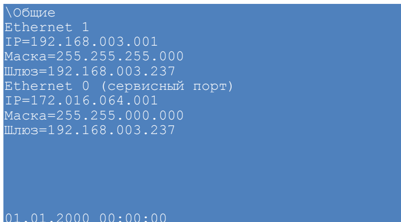
Рисунок 33 – Внешний вид пункта меню Общие
